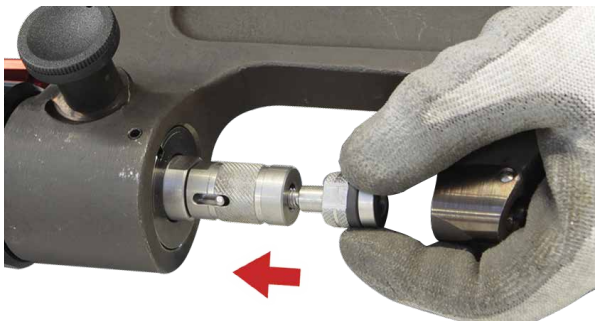
パンチ/マンドレルサポート
